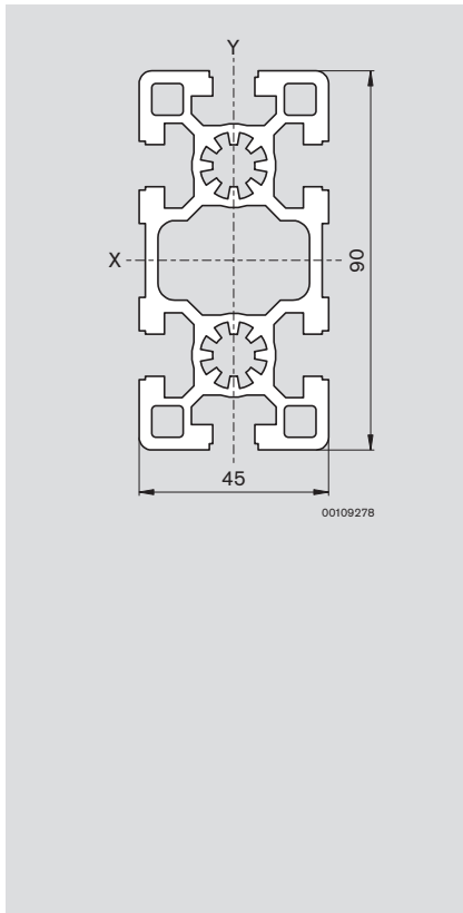
45x90
