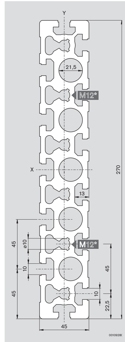
45x270
